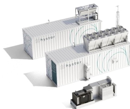
ハイスター社の水電解装置
